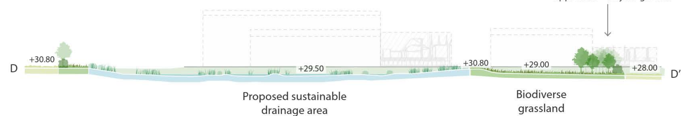
Section D - D'
